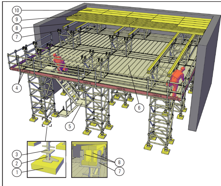
Figur A. Beskriver formställning och form som används vid valv i byggnad
